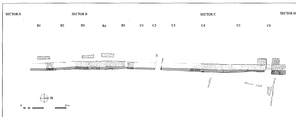
Planta general de la primera muralla ibèrica, bastida entre les darreries del segle V i començaments del IV a.C., on es pot veure, assenyalat amb una trama, el reforç de la cara externa, aixecat cap a mitjans del segle IV a.C.
