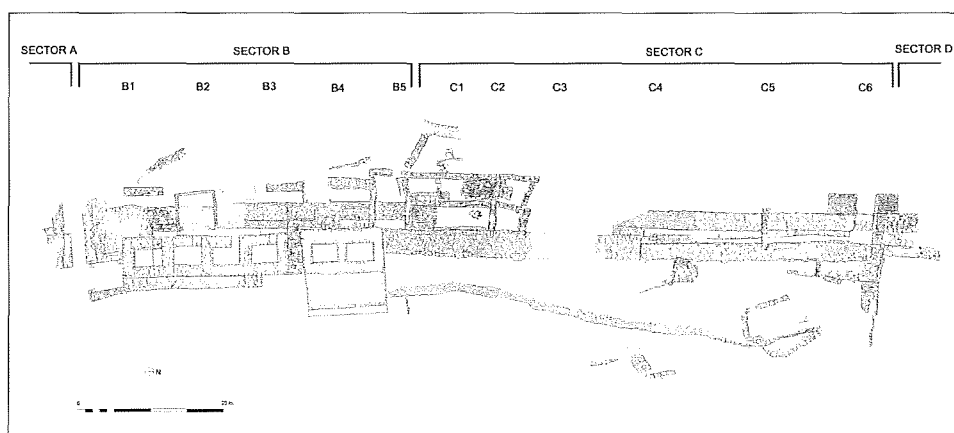
Planta general del conjunt arqueològic del Montgròs amb la nomenclatura assignada als diversos sectors.
