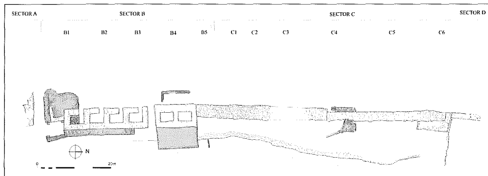
Planta general de la muralla ibèrica principal, amb els primers reforços que s'hi van fer en el decurs del segle III a.C.: construcció dels bastions 1 i 2, reforçament de la porta amb una torre interior i aixecament d'un parament extern adossat als sectors B1 i B2 de la muralla.
