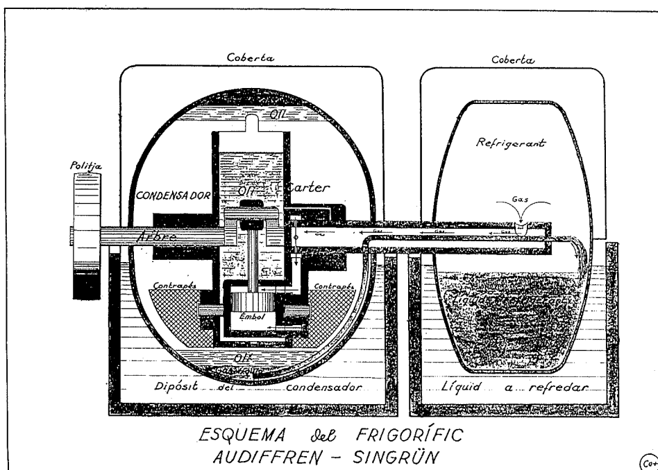
Fig. 1. Màquina de refredar.
